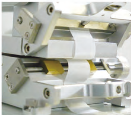
柔性磨擦设置 (标配)
