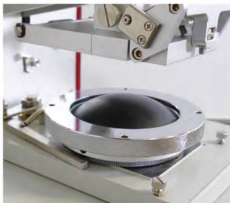
充气隔膜设置 (标配)
