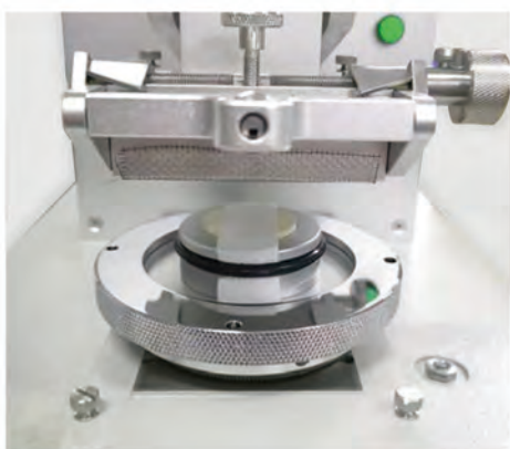
平磨附件和弹性垫/磨擦设置 (可选)
