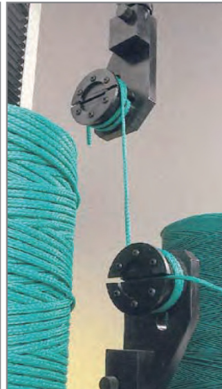
细线/绳索测试
