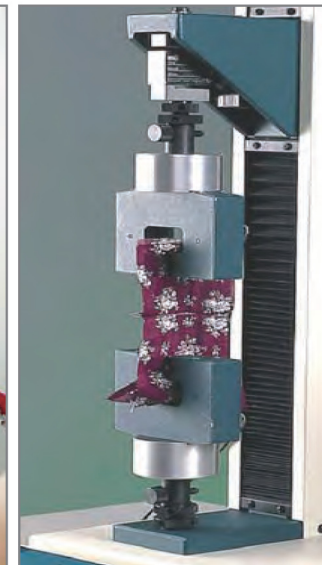
使用气动夹具进行 接缝打滑测试
